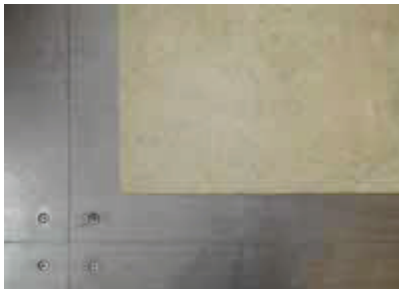
Figure 1 : Emplacement d'une dalle de 450 x 450 mm, qui doit être décalée de 75 mm de chaque bord d'un panneau de plancher surélevé.
