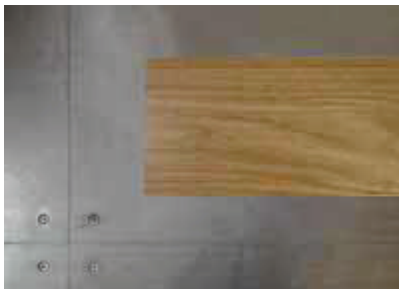
Figure 2 : Emplacement d'une lame de 1000 x 150 mm, qui doit être décalée de 75 mm et de 100 mm des bords d'un panneau de plancher surélevé.
